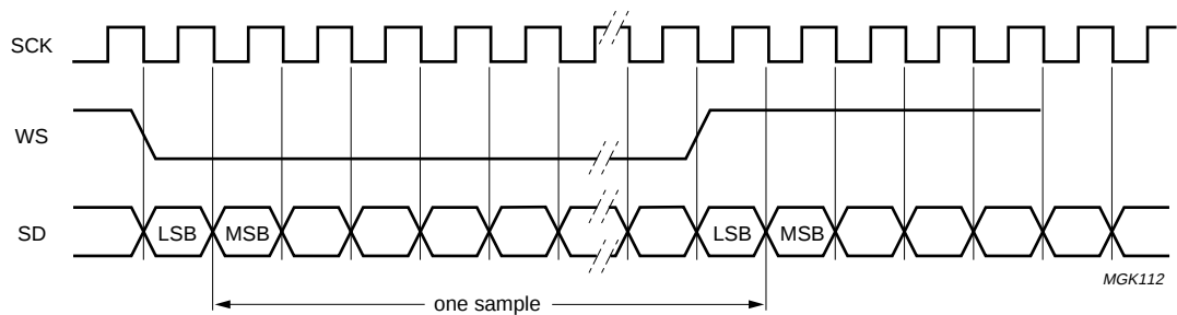
a. I²S-bus format.
