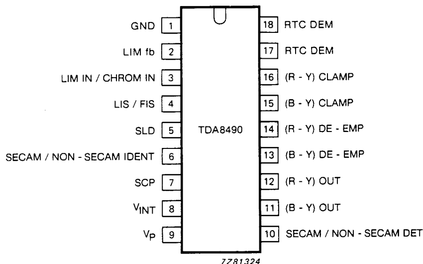
Fig. 2 Pinning diagram.
