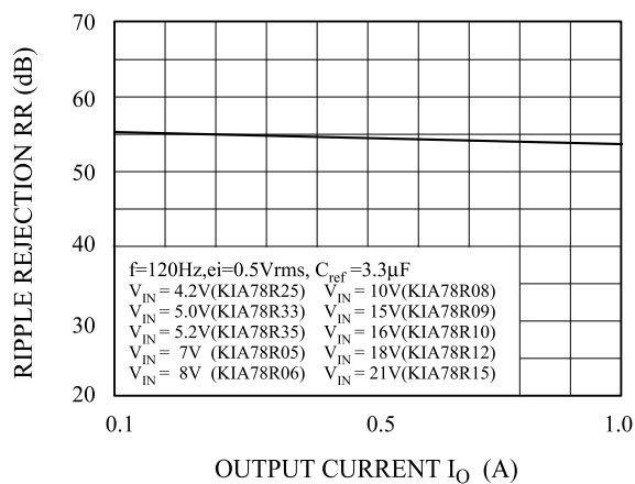
Fig. 10 R.R - I_{OUT}
